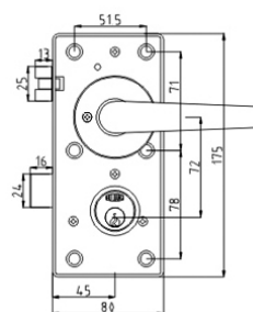
C2-B чертёж
