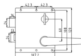
C2 чертёж
